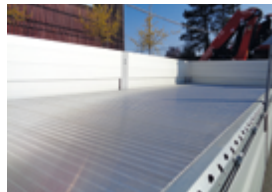
Ladungssicherung NK-Fix
